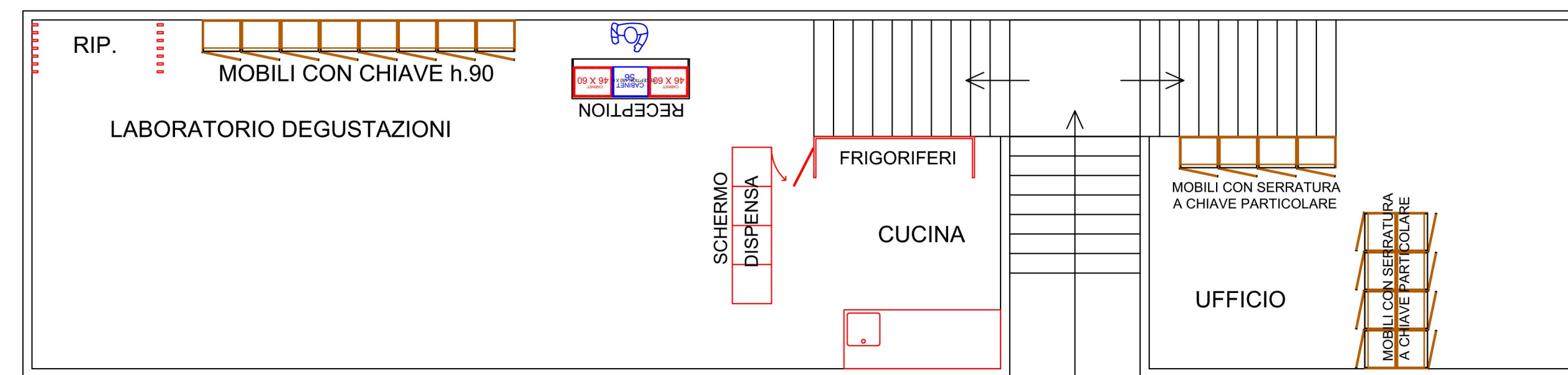
PLANIMETRIA PIANO PRIMO SOPPALCO PIANO 1°
